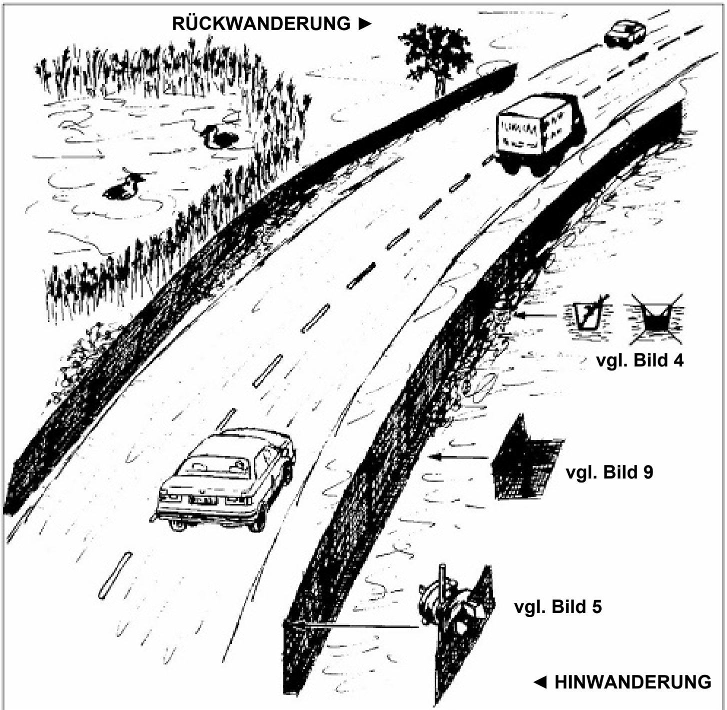
Bild 2: SCHWEGLER Amphibienschutzzaun (detailliertes Aufstellungsschema)
